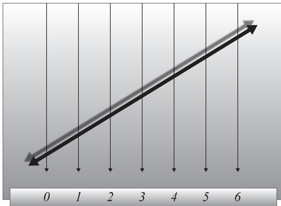
Figura 1: Scala Kinsey
